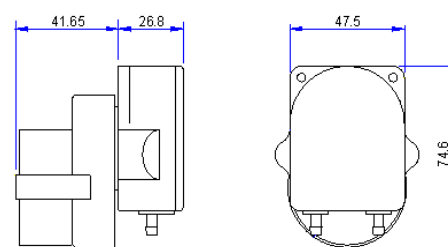
Moteur synchrone
