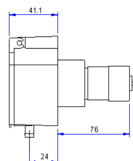
Côtes d'encombrement en mm
