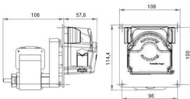
Côtes d'encombrement en mm
