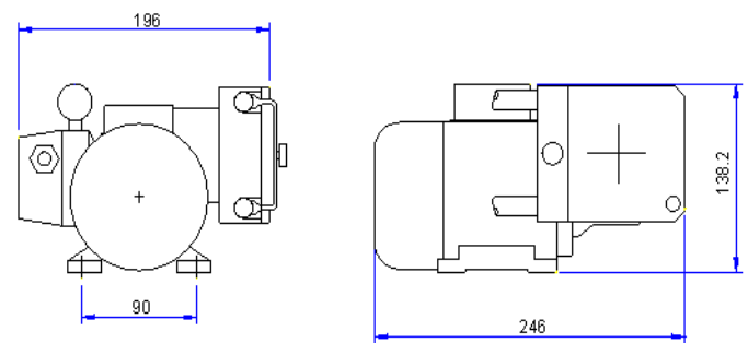
Côtes d'encombrement en mm. ( moteur 230 V 50 Hz IP55 )
